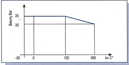
Grafik 1 : Basınç - sıcaklık ilişkisi Nota : 1 bar = 10 5 N/m 2 = 100kPa
